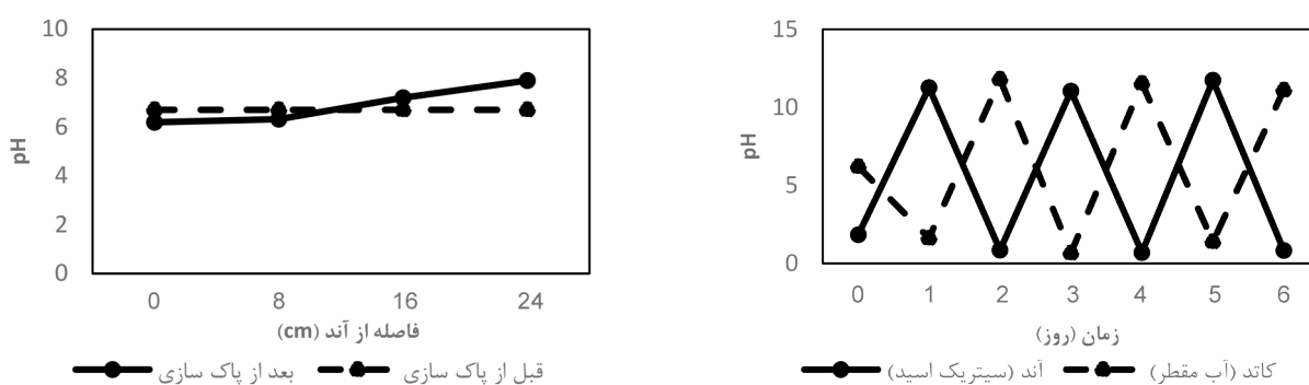
نمودار ۲- (الف) تغییرات pH مخازن؛ (ب) تغییرات pH خاک؛ در راکتور EK6 با تعویض قطبیت
