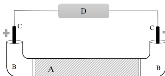
شکل ۱- شماتیک راکتور مورد استفاده (A: محیط آلوده؛ B: مخزن الکترولیت؛ C: الکتروود؛ D: منبع تغذیه)
