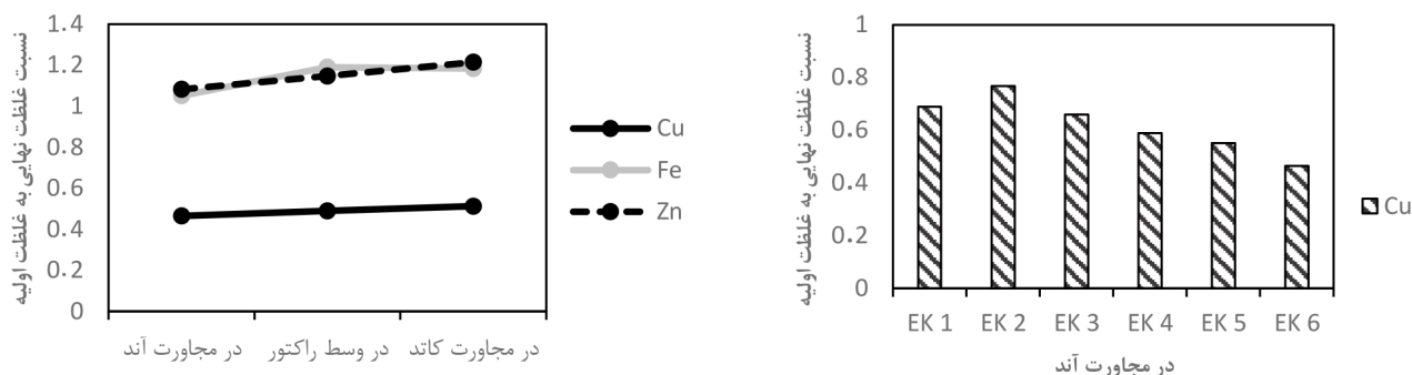
نمودار ۱- (الف) غلظت فلز سنگین مس در راکتورها؛ (ب) غلظت فلزات مس، آهن و روی در حالت بهینه (راکتور EK6)
